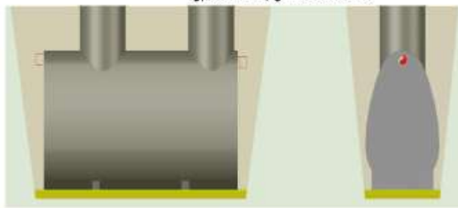
Монтаж вне пределов проезжей части с низким уровнем грунтовых вод.
