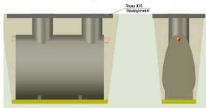
Монтаж в пределах проезжей части
