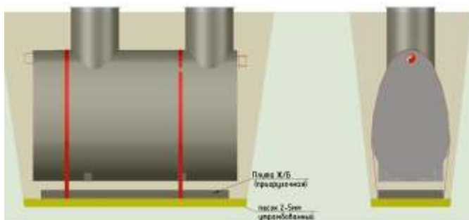
Монтаж в пределах проезжей части
