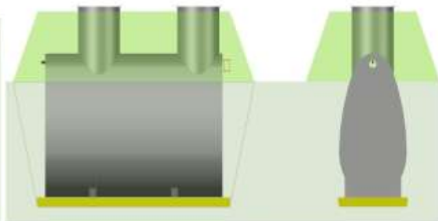
Монтаж вне пределов проезжей части с низким уровнем грунтовых вод.
